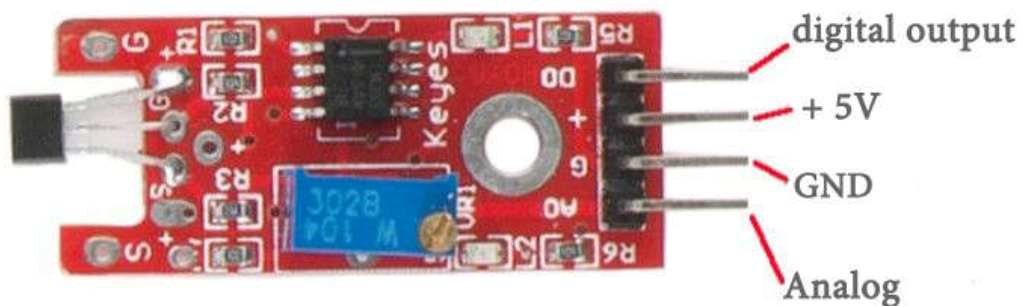
Linear Hall
